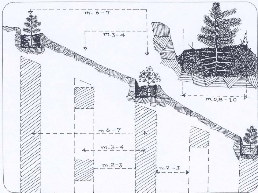
Fig. 1. Schematizzazione del tipo di lavorazione misto a trincee e a buche. Sezione e prospetto degli interventi in superficie.
