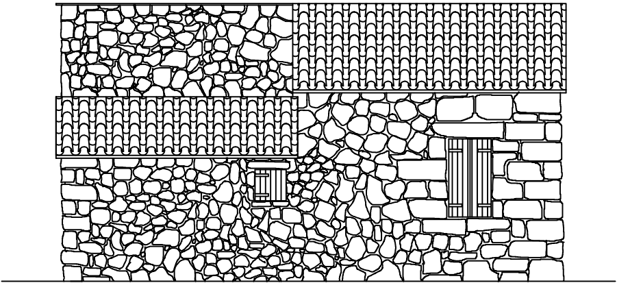
PROSPETTO D
