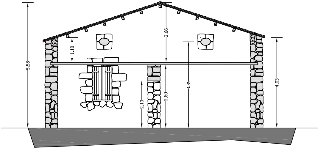
SEZIONE
