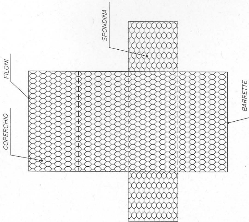
GABBIONE APERTO
